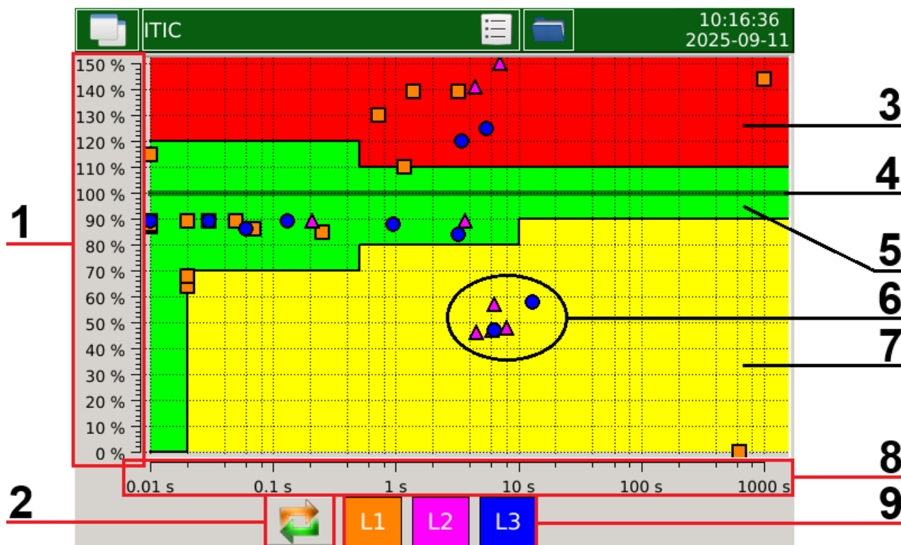
Rys. 2.3.3.11.1. Krzywa ITIC.
