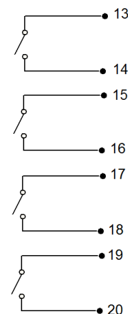
Rys. 13. Wyjścia przekaźnikowe.
