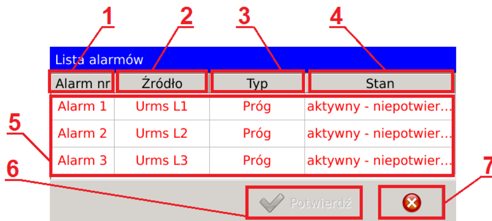
Rys. 168. Alarmy - lista alarmów, opis.
