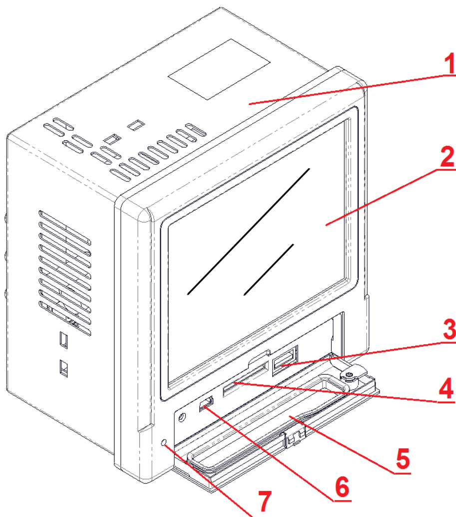
Rys. 173. Budowa ND45PLUS.
