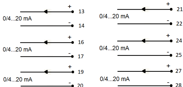
Rys.17. Wyjścia analogowe.
