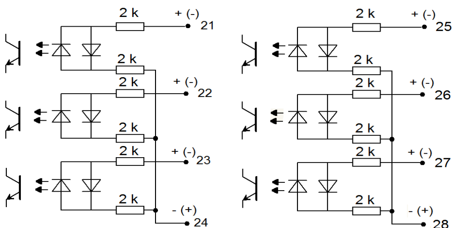
Rys. 16. Wejścia binarne.
