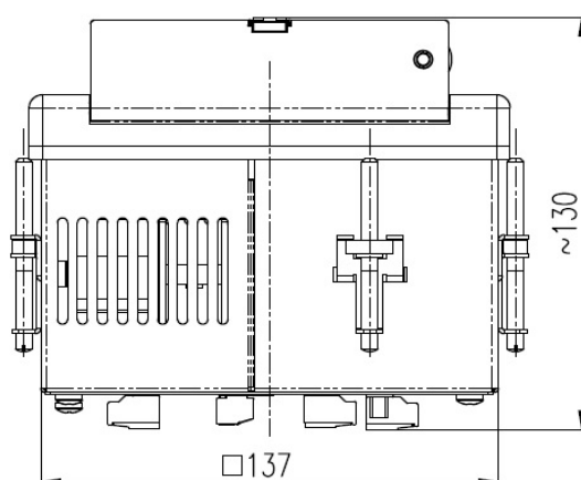
Rys. 20. Wymiary - dół.
