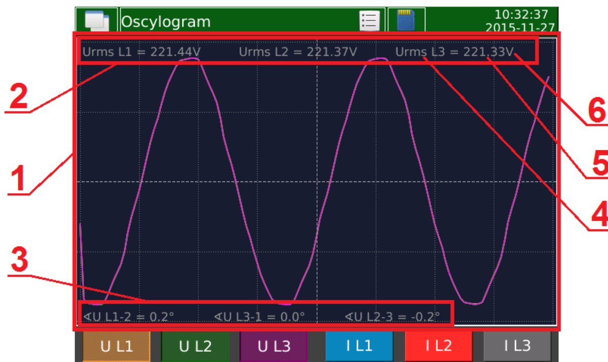
Rys. 74. Oscylogram.
