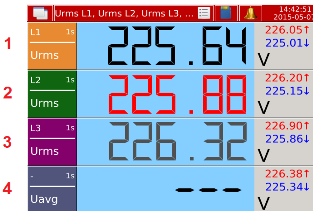
Rys. 57. Prezentacja danych pomiarowych.
