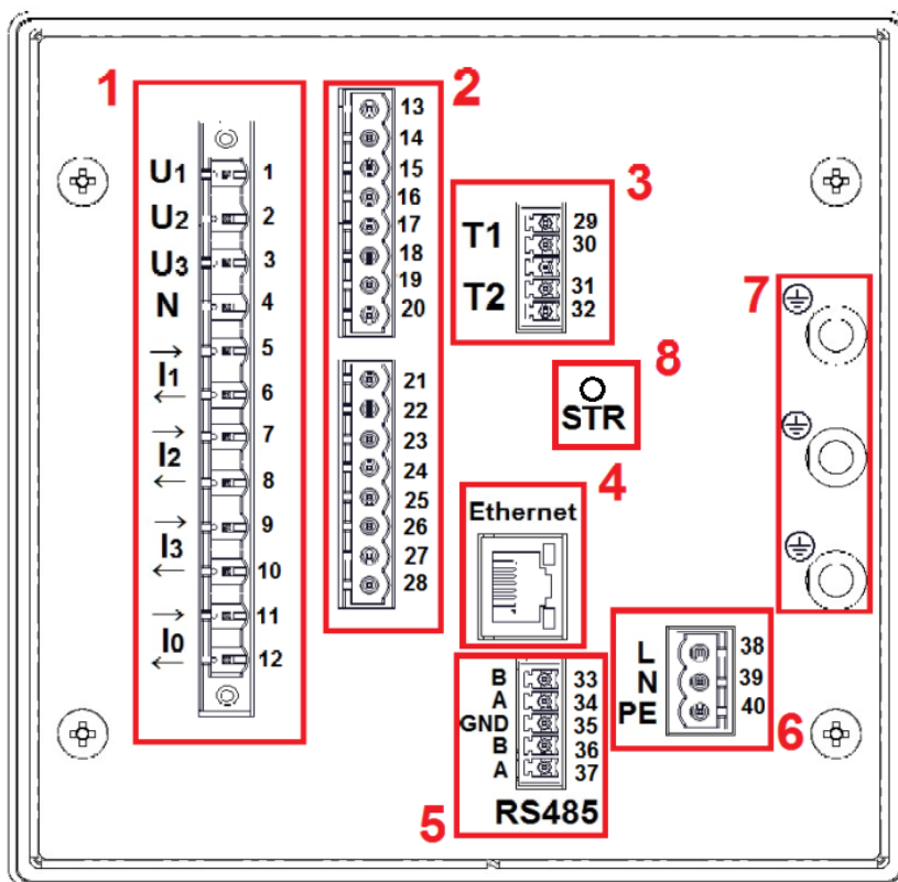
Rys.1. Płyta zaciskowa.
