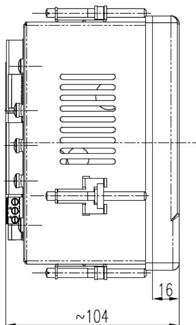
Rys. 22. Wymiary - bok.
