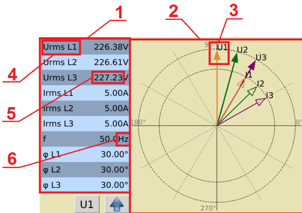
Rys. 73. Diagramy wektorowe.
