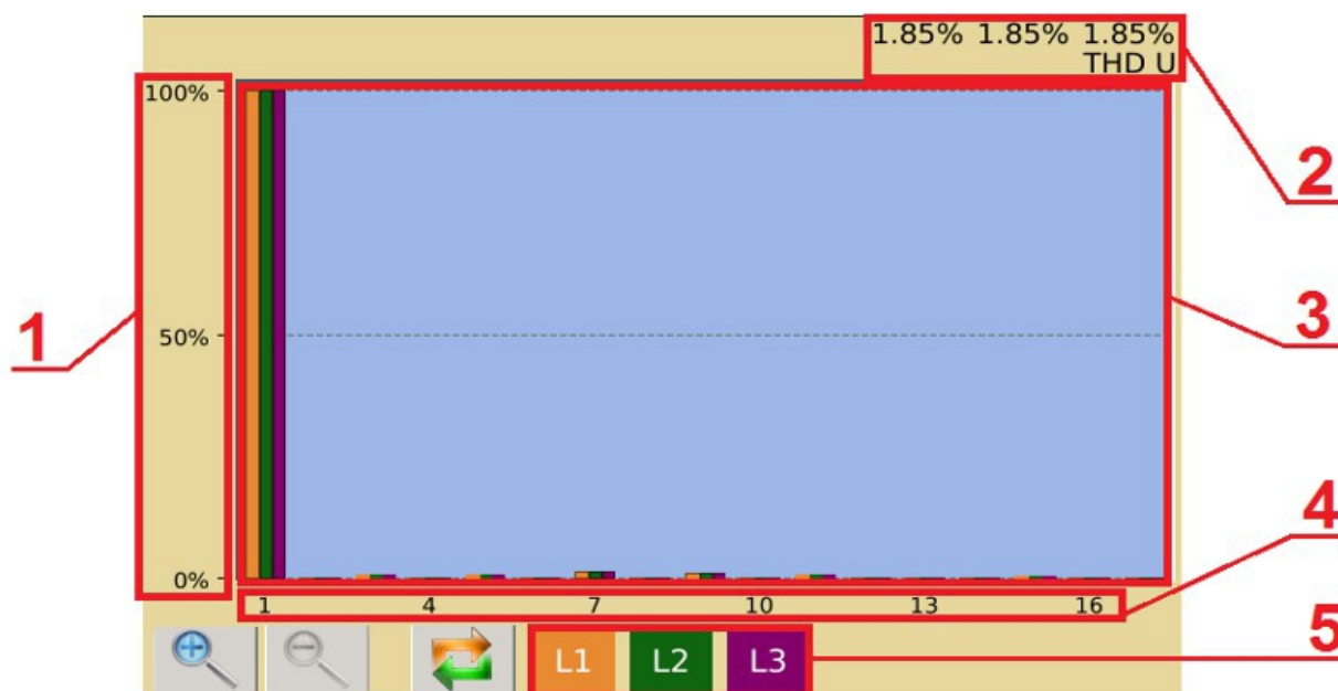
Rys. 68. Harmoniczne.
