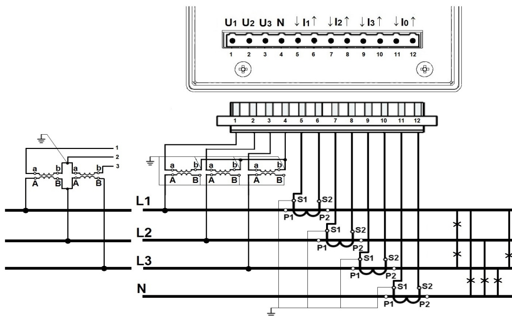
Rys. 9. Schemat - sieć czteroprzewodowa.
