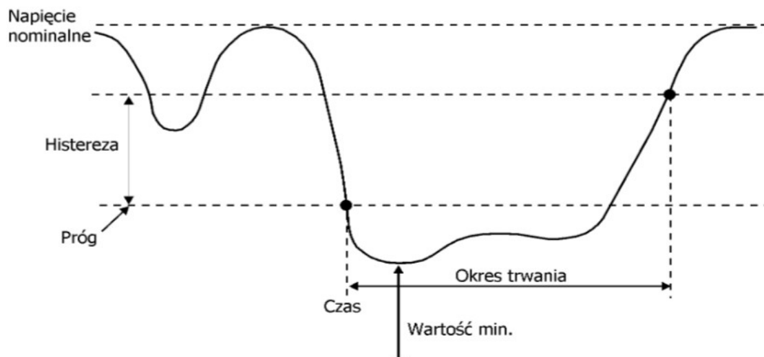
Rys.149. Zapad napięcia.
