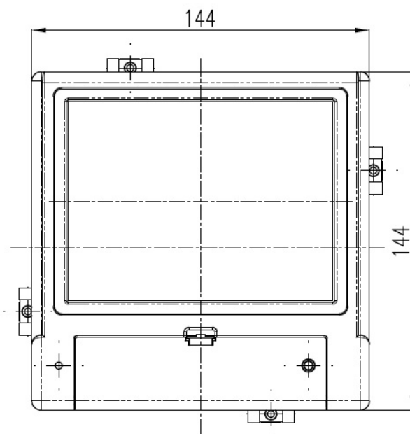
Rys. 21. Wymiary - przód.
