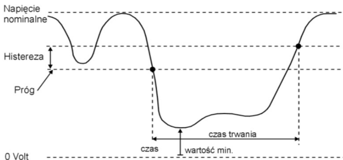
Rys.151. Zanik napięcia.
